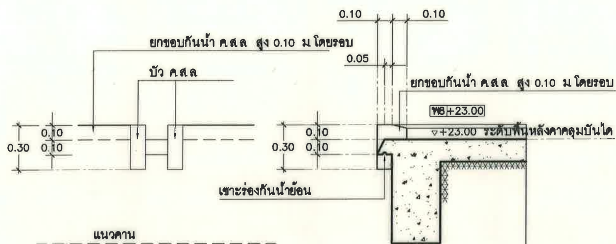
แบบขยายขอบวางน้ำ ค.ส.ล
