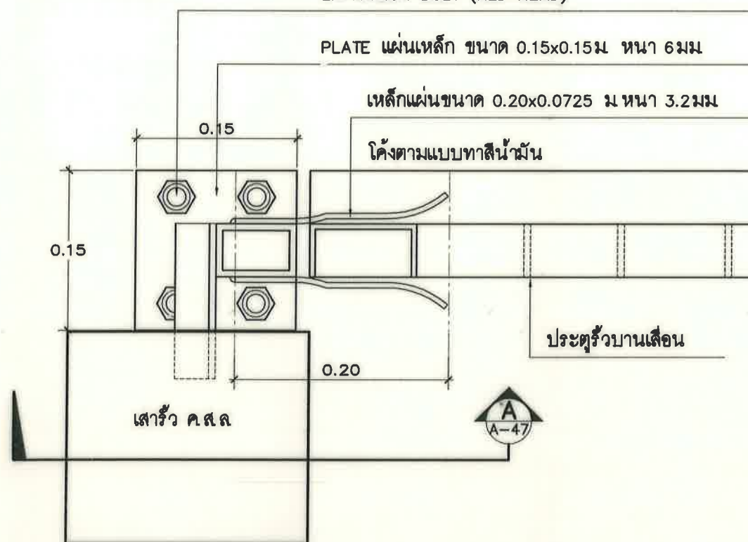
แปลนแบบขยายเสาเหล็ก กันชนประตูลูกบิดเลื่อน มาตราส่วน 1 : 5
