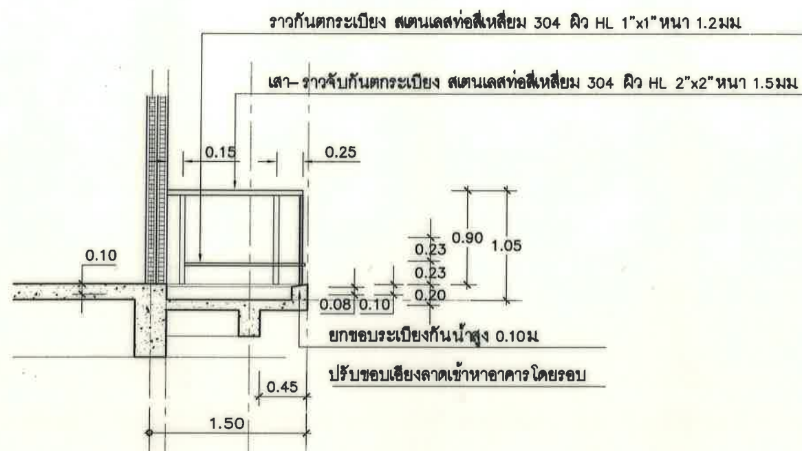
รูปตัดขยายระเบียง มาตราส่วน 1 : 50
