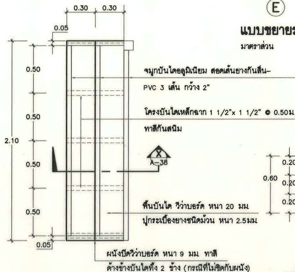
แปลนขยายบันไดต่างระดับภายใน
