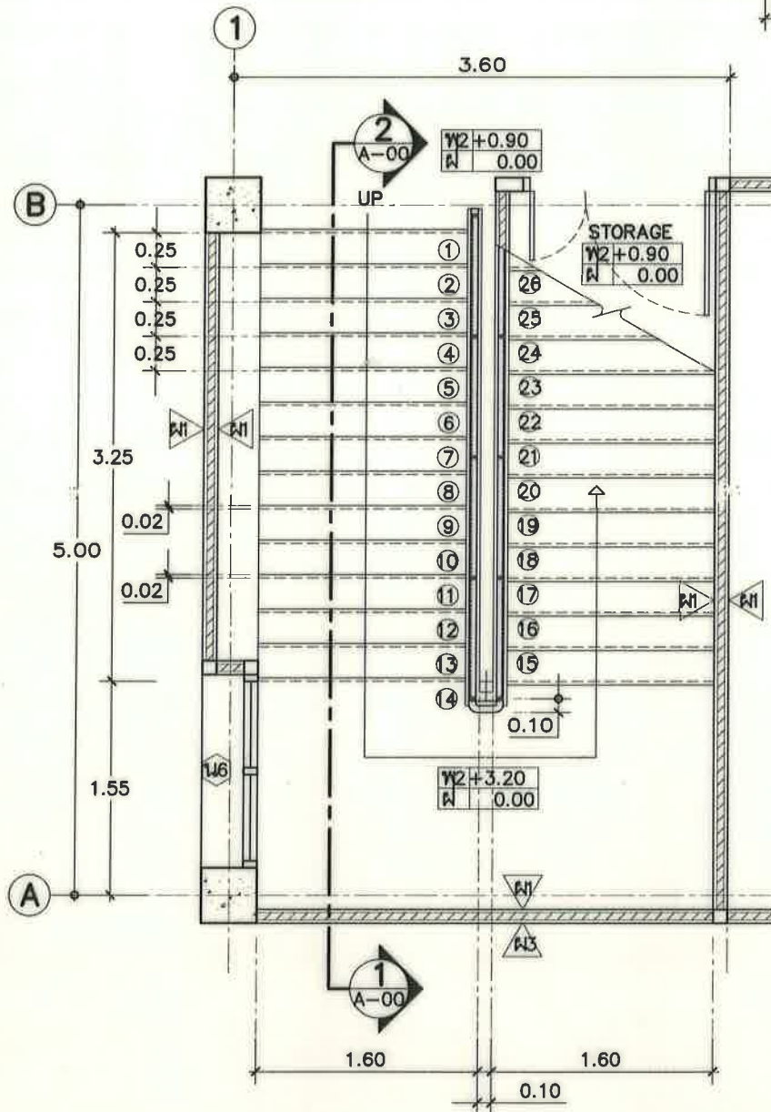
แปลนขยายบันไดชั้น 1 ST-2 มาตราส่วน 1 : 50
