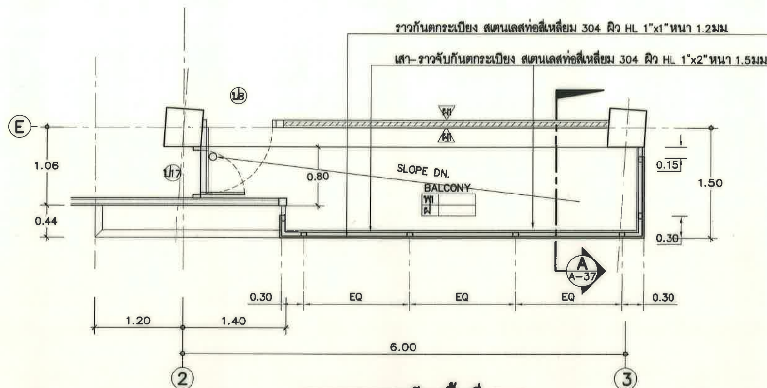
แบบขยายระเบียงชั้นที่ 3-4 มาตราส่วน 1 : 50
