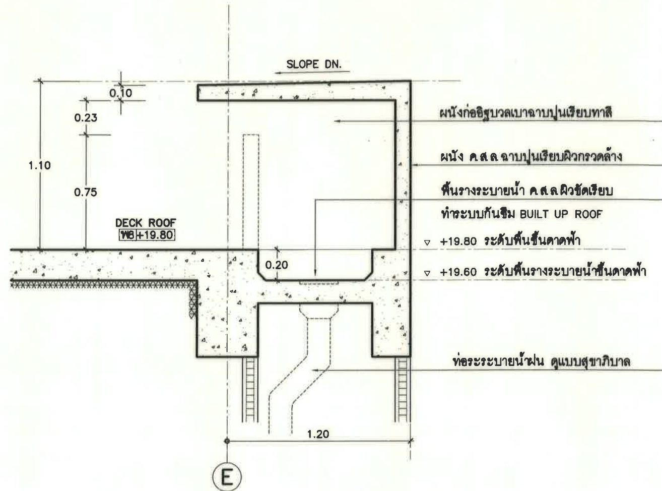
แบบขยายวางระบายน้ำชั้นดาดฟ้า
