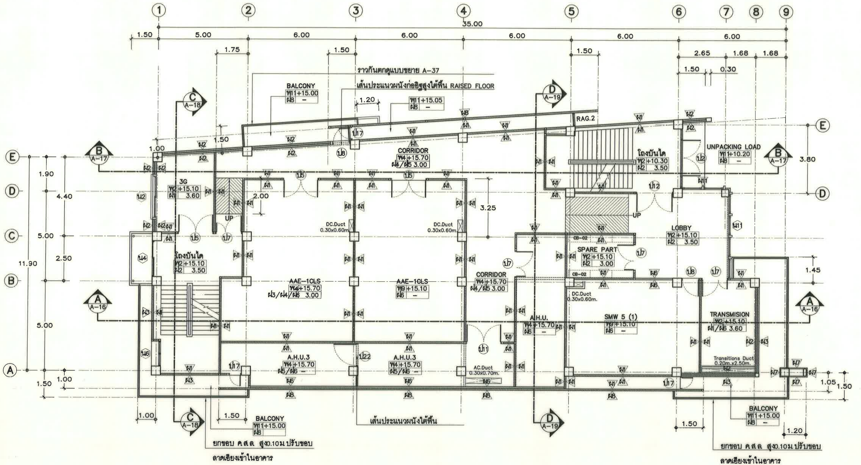
แปลนพื้นที่ 4 มาตราส่วน 1 : 125
