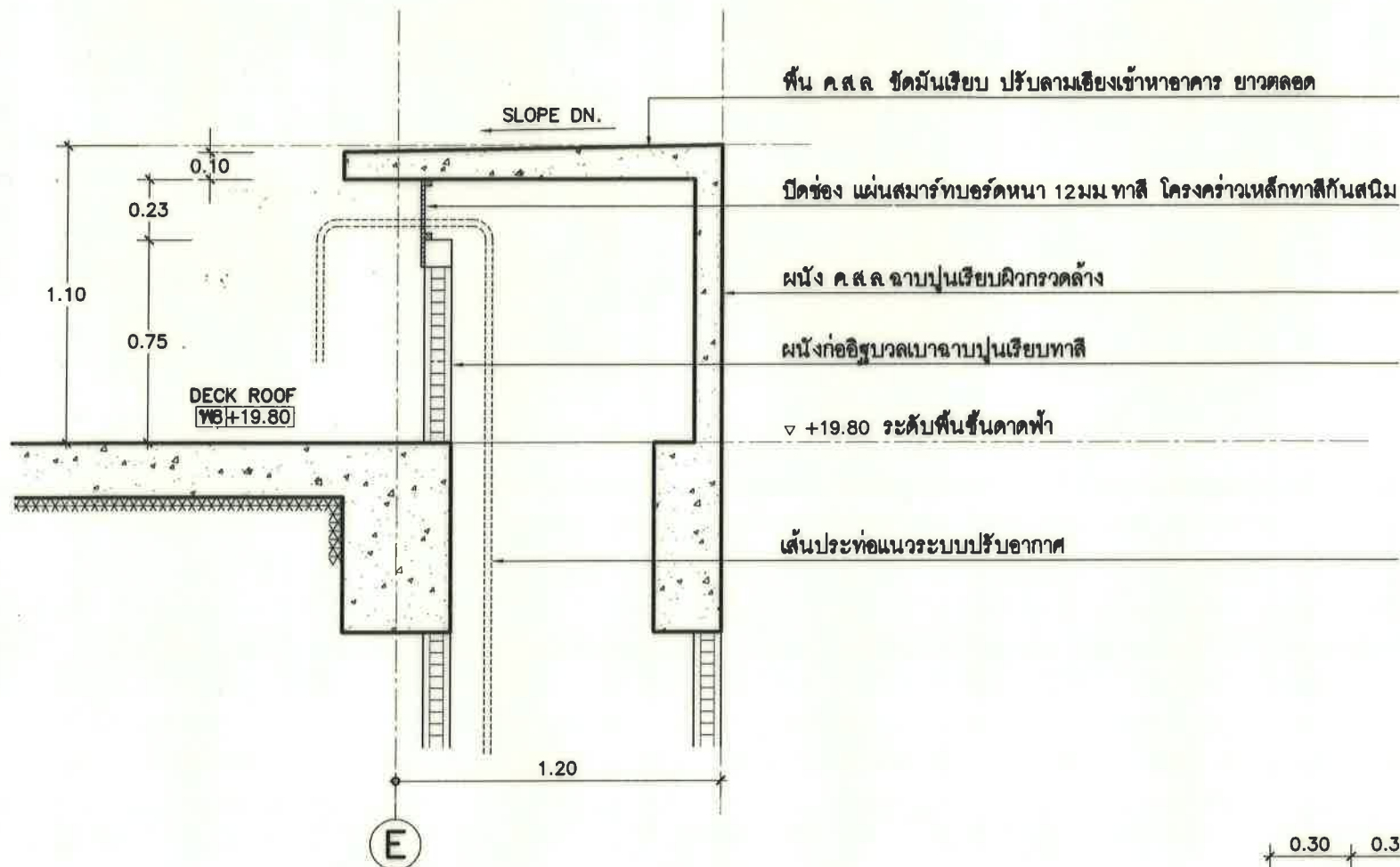
แบบขยายช่อง DUCT แอร์ ชั้นดาดฟ้า
