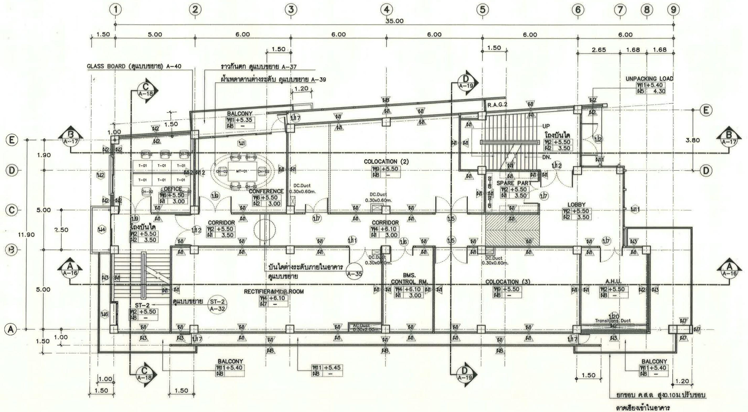
แปลนพื้นที่ 2 มาตราส่วน 1 : 125
