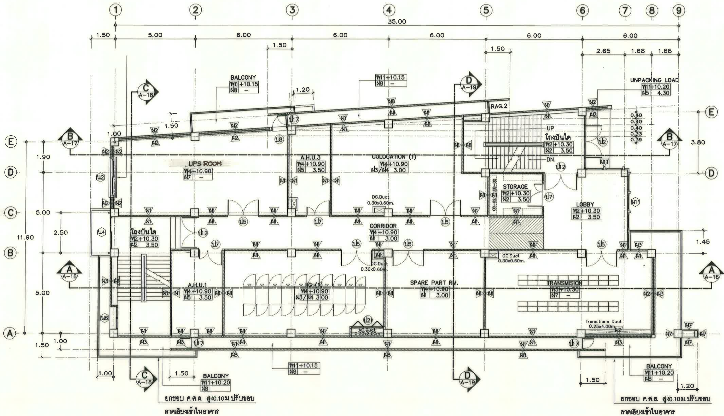
แปลนพื้นที่ 3 มาตราส่วน 1 : 125
