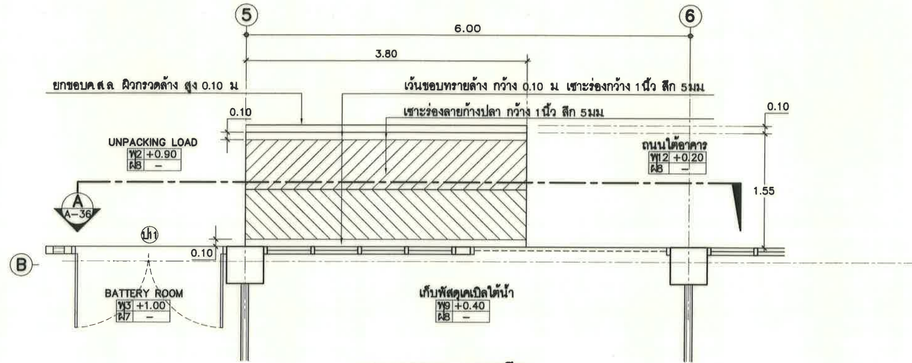
แบบขยายทางลาดเอียง
