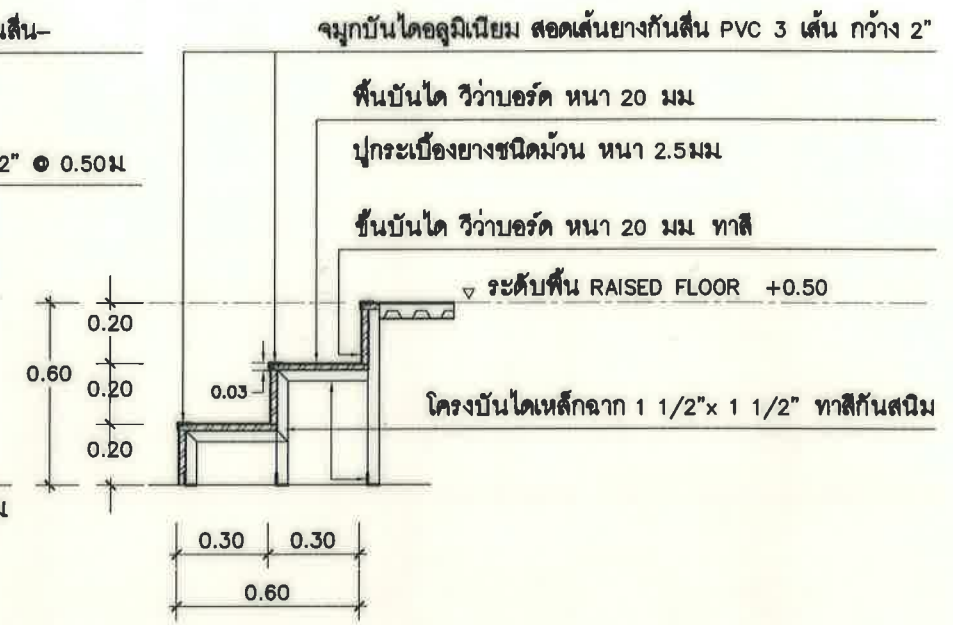
รูปตัดขยายบันได
