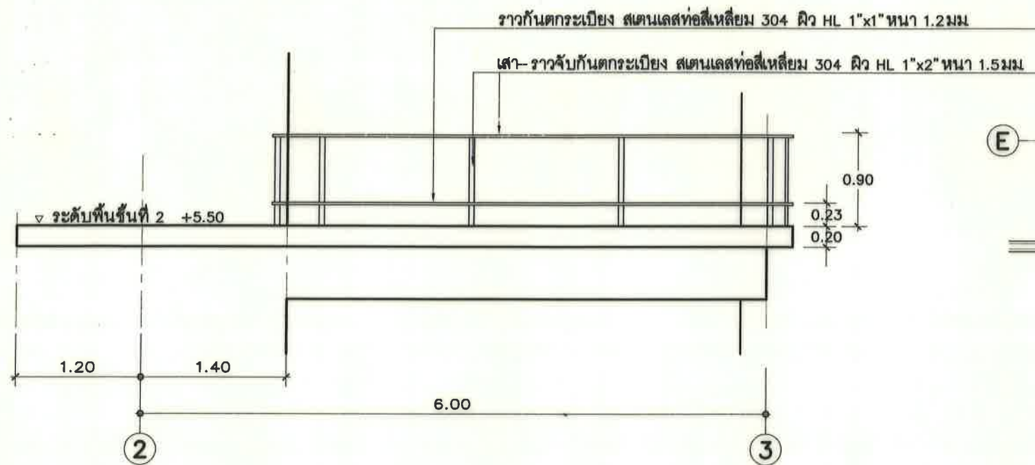
รูปด้านขยายระเบียง มาตราส่วน 1 : 50
