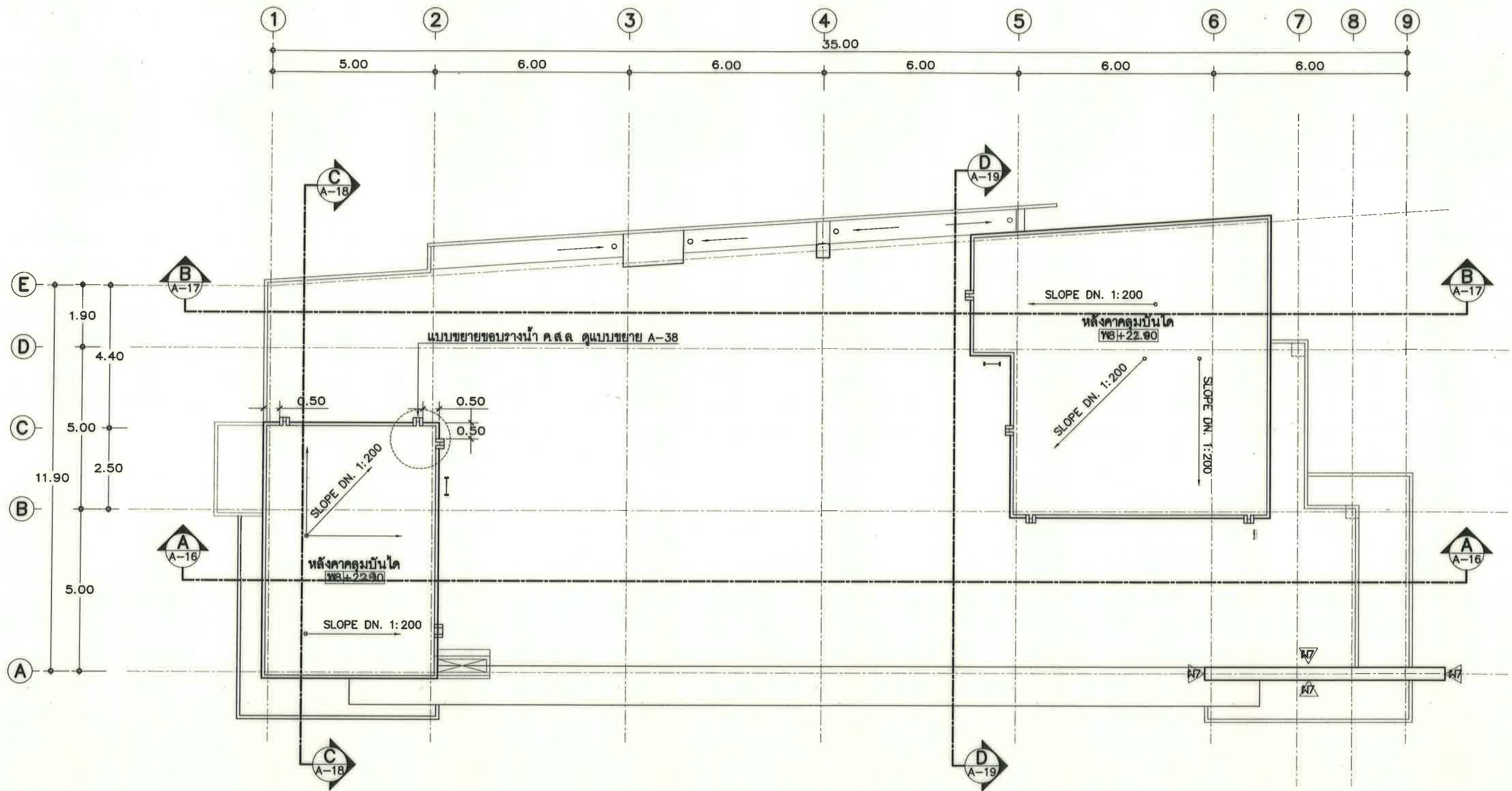
แปลนพื้นหลังคาคลุมบันได มาตราส่วน 1 : 125
