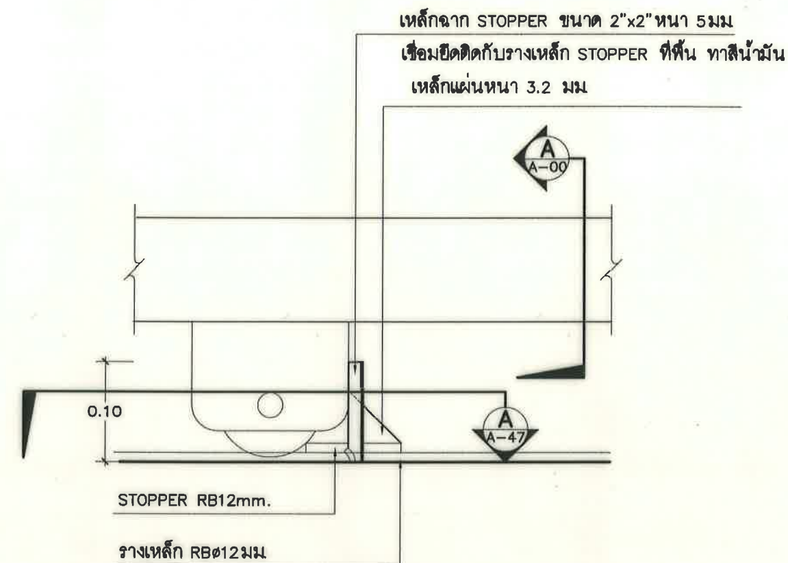
แปลนแบบขยายSTOPPER ประตูลูกบิดเลื่อน มาตราส่วน 1 : 5
