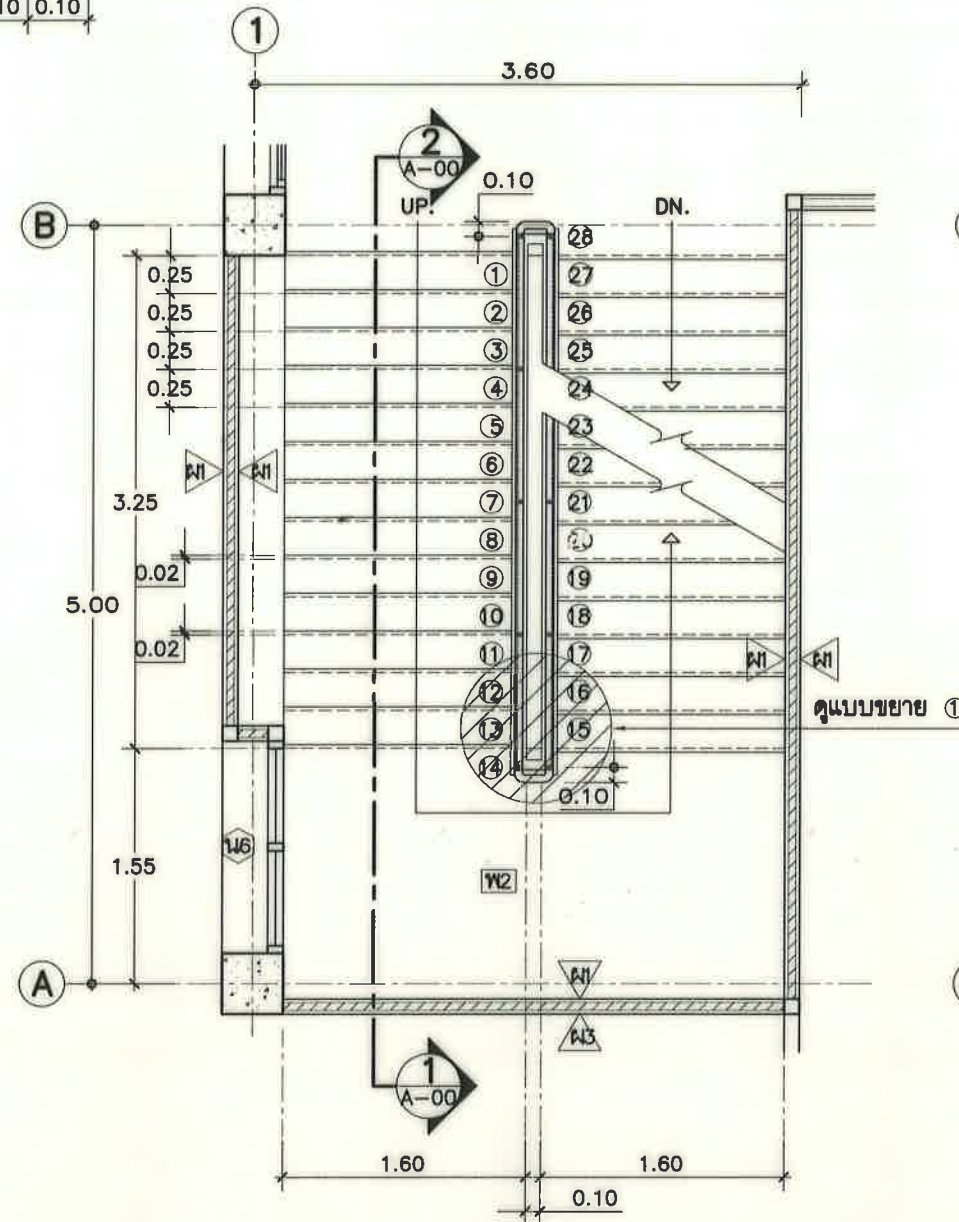
แปลนขยายบันไดชั้น 2-4 ST-2 มาตราส่วน 1 : 50
