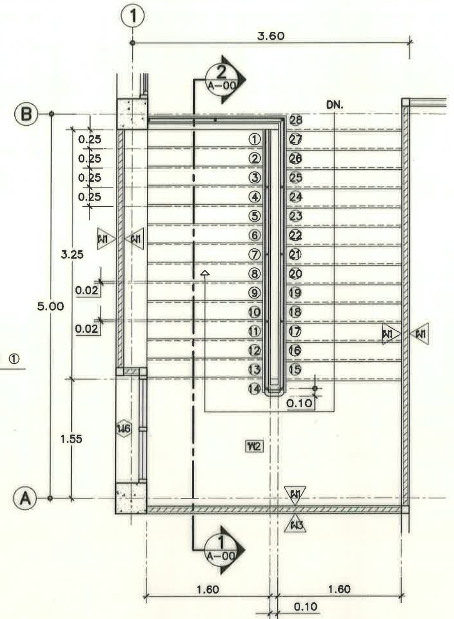
แปลนขยายบันไดชั้นดาดฟ้า ST-2 มาตราส่วน 1 : 50
