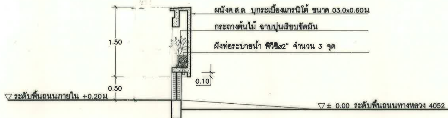
แสดงแนวตัด X มาตราส่วน 1 : 50
