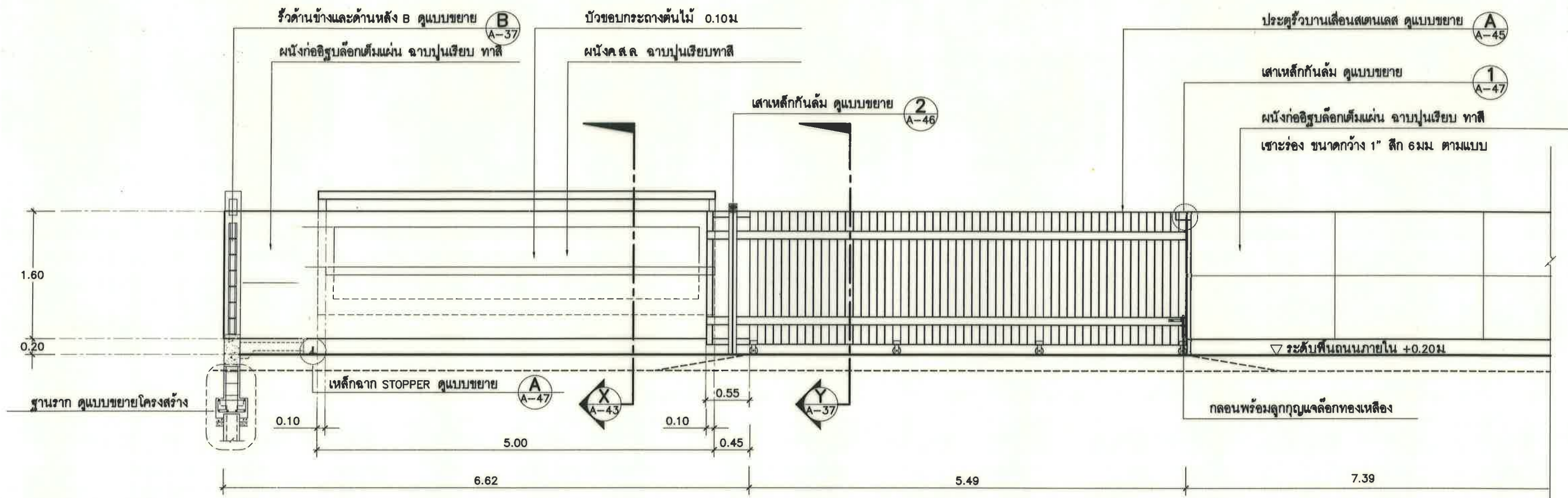
แสดงรูปด้าน 2 มาตราส่วน 1 : 50
