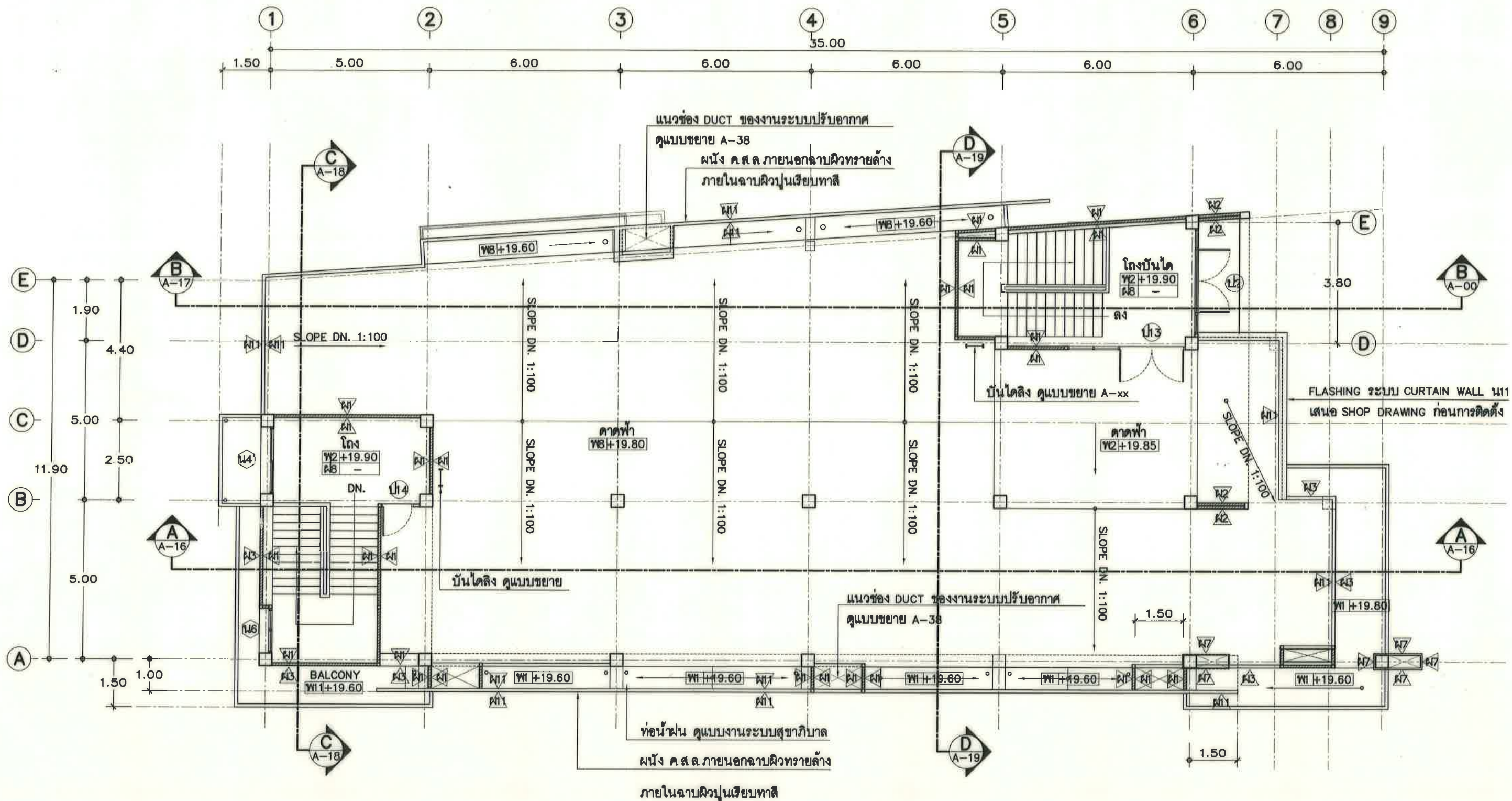
แปลนพื้นชั้นคาเฟ่ มาตราส่วน 1 : 125
